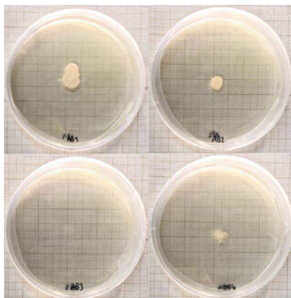
Figure 14 Visuel des 4 éprouvettes d' Aspergillus niger exposées aux vapeurs d'eau-butanol à J8. © Mathilde Bezon.
